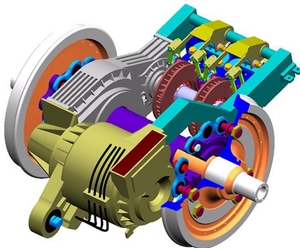
Lokomotivní dvojkolí
